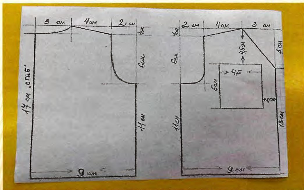
ВЫКРОЙКА ЖИЛЕТА МАСШТАБ 1:1
